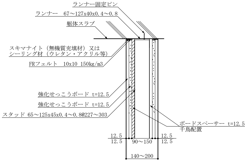
断面詳細図
