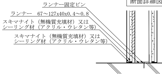
断面詳細図
