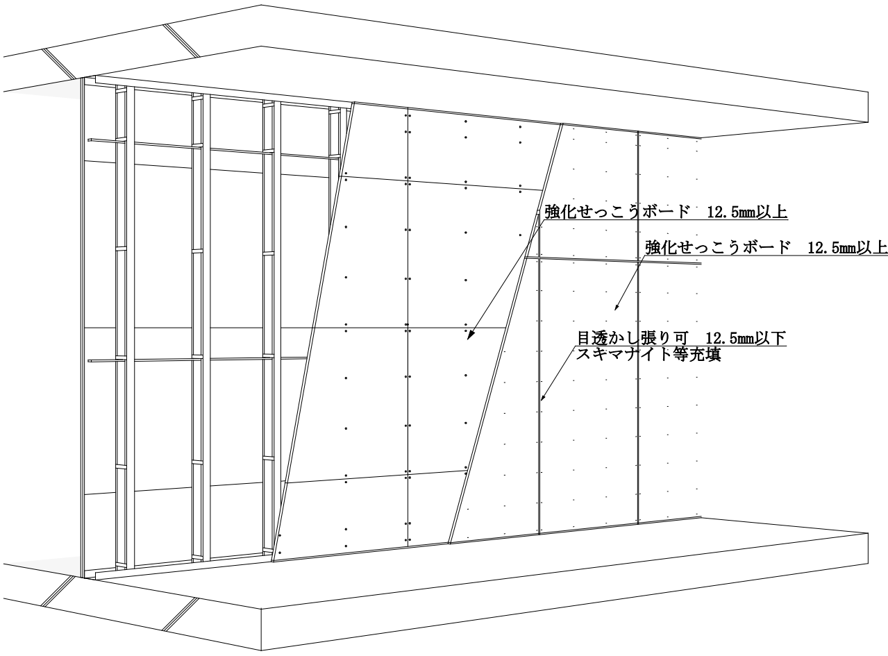
目すかし部処理方法（例）
