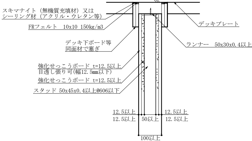
デッキ（床躯体）取合い（直交） 断面詳細
