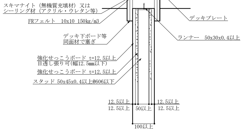
デッキ (床躯体) 取合い (直交) 断面詳細
