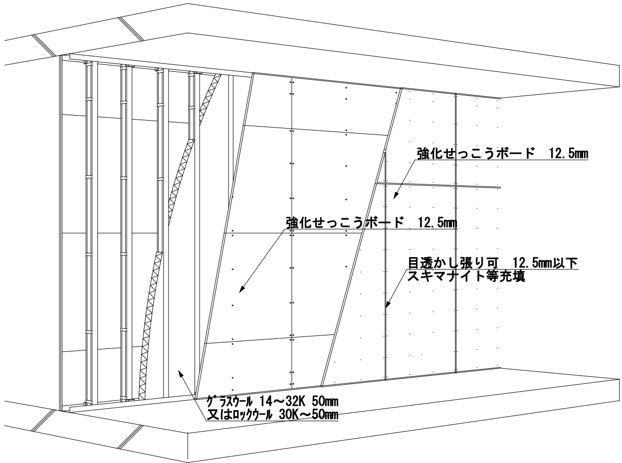
目すかし部処理方法（例）
