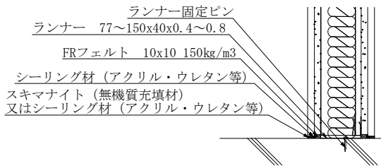
断面詳細図
