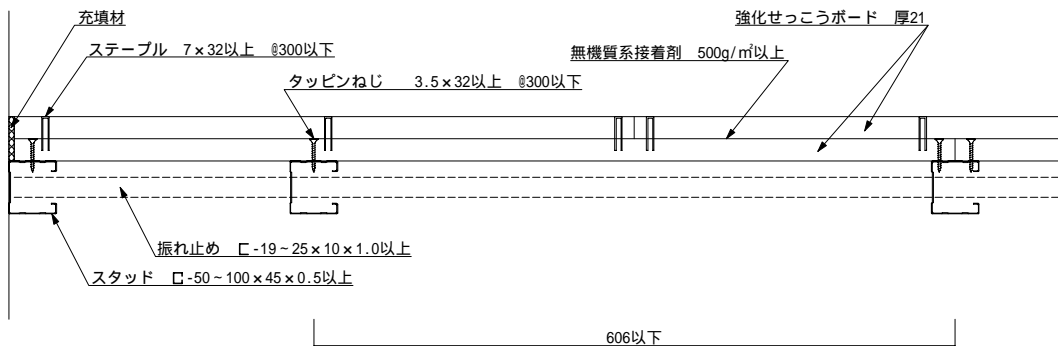
鉛直断面図
