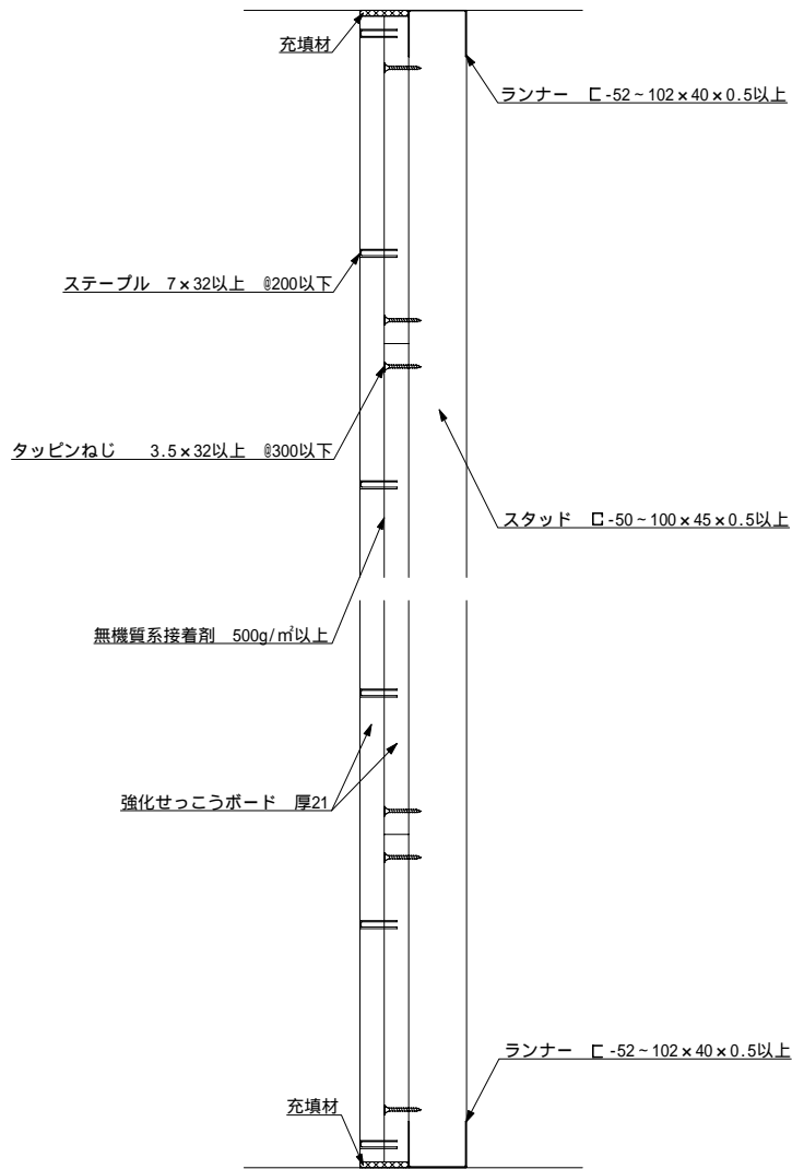
水平断面図
